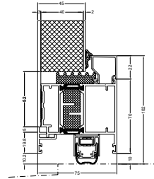
PANNEAU POUR PORTE À OUVRANT CACHÉ
